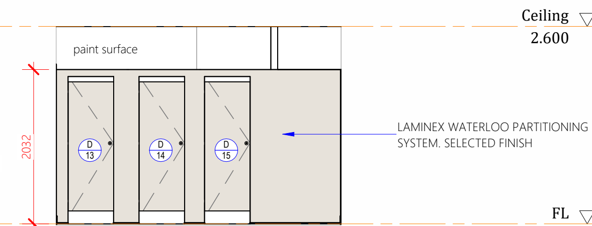
Elevation 4E 1 : 50
