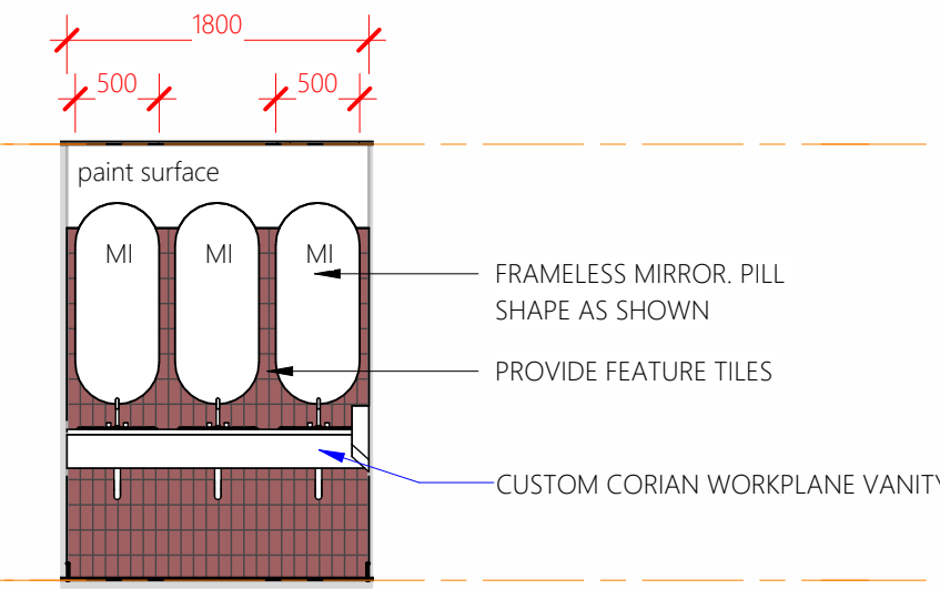
Elevation 3B
