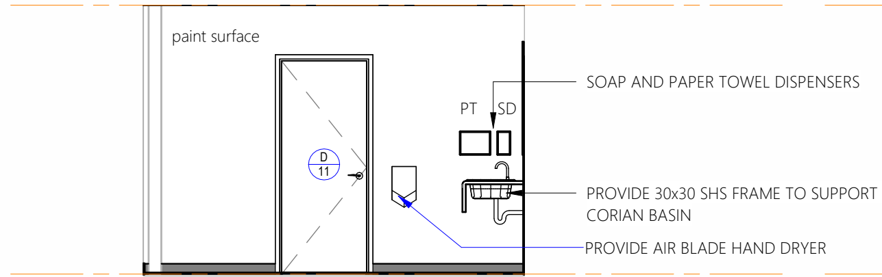
Elevation 4D 1 : 50
