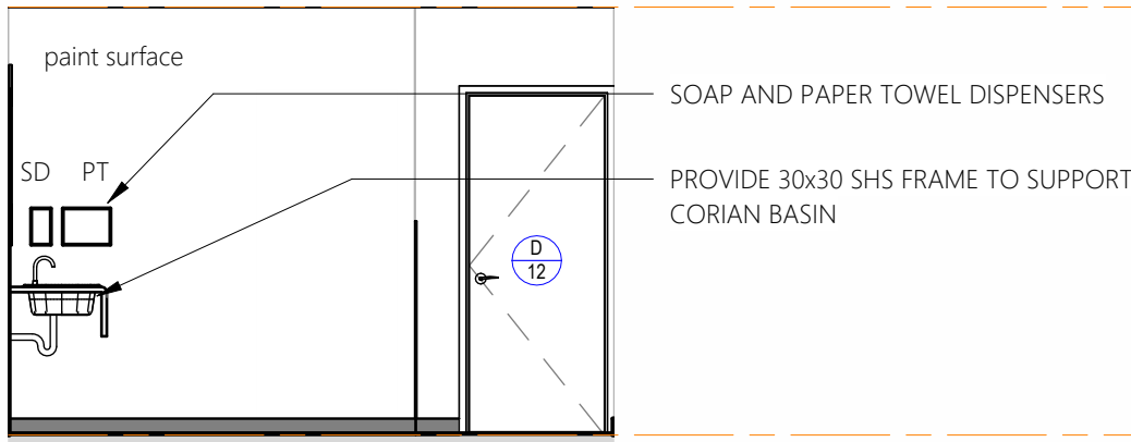
Elevation 4B 1 : 50
