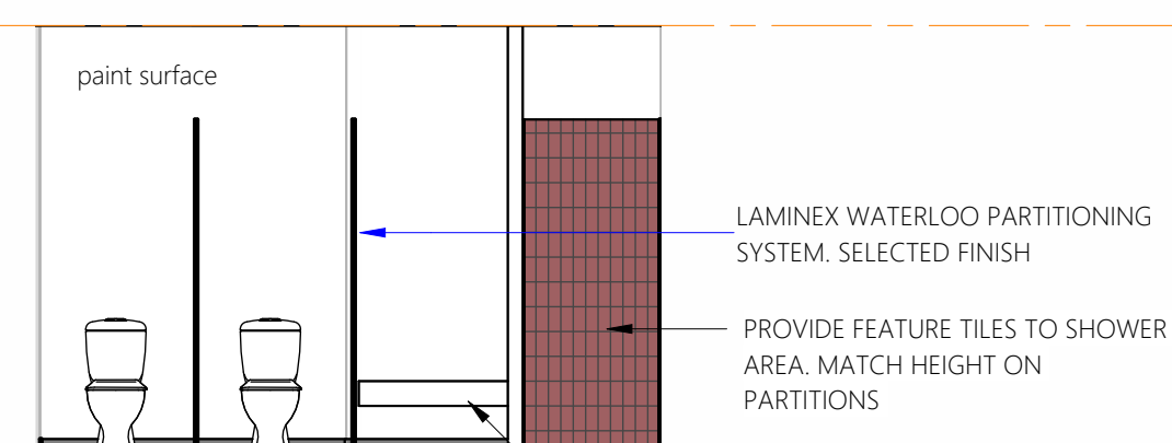
Elevation 4I 1 : 50
