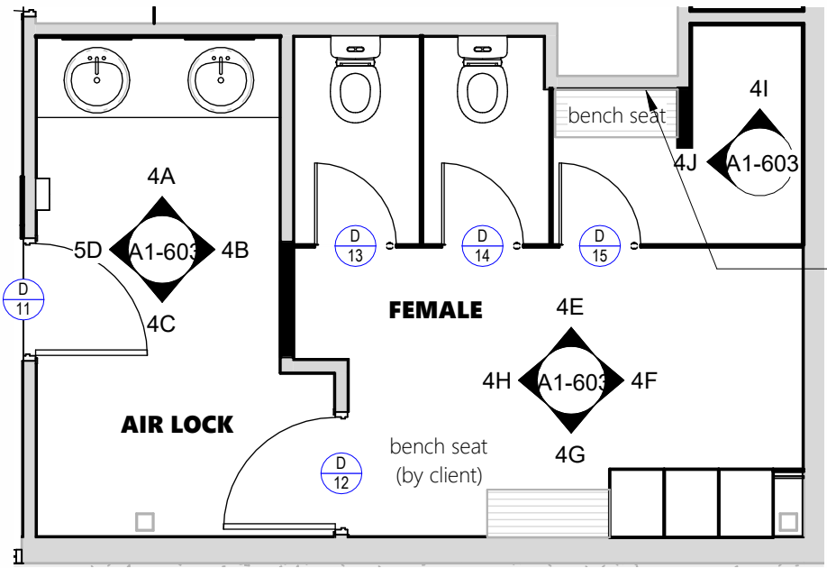
Internal Plan 4 1 : 50
