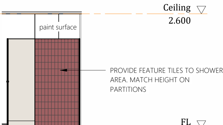
Elevation 4J 1 : 50
