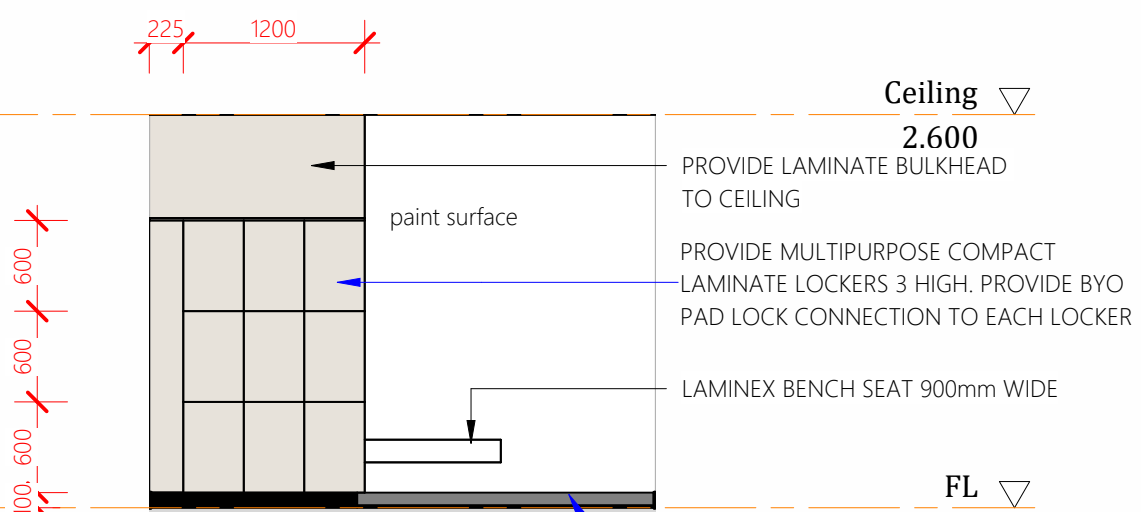
Elevation 4G 1 : 50
