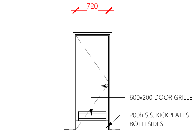
DOOR TYPE D
