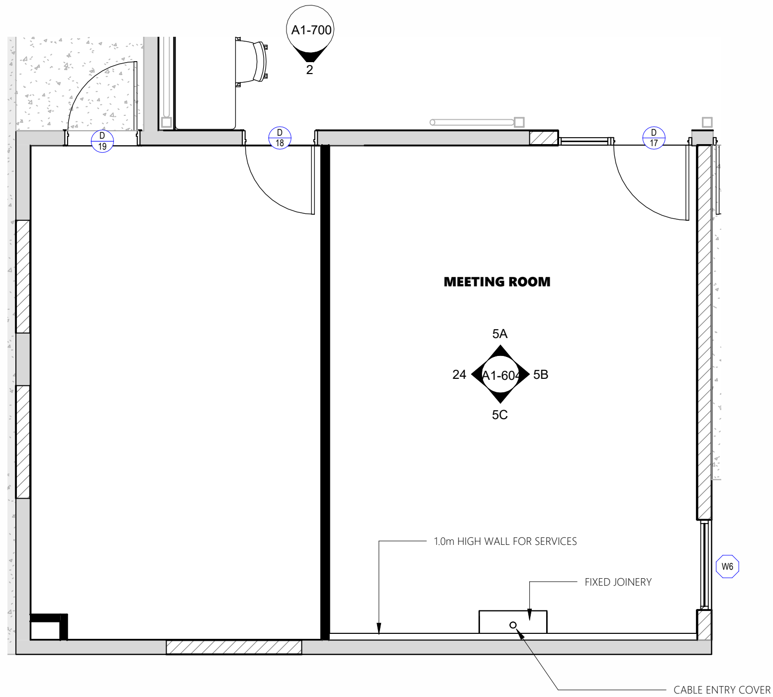
Internal Plan 5 1 : 50
