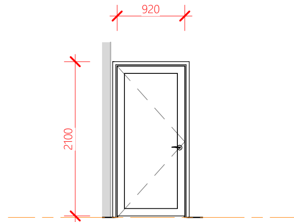
DOOR TYPE H
