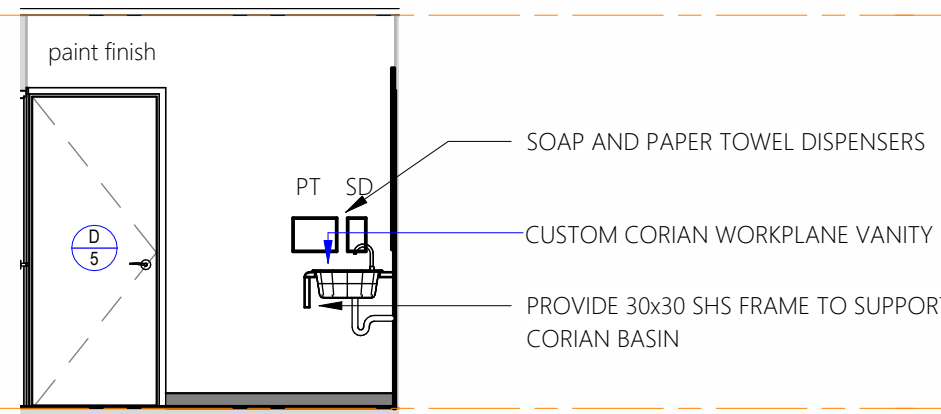
Elevation 3E
