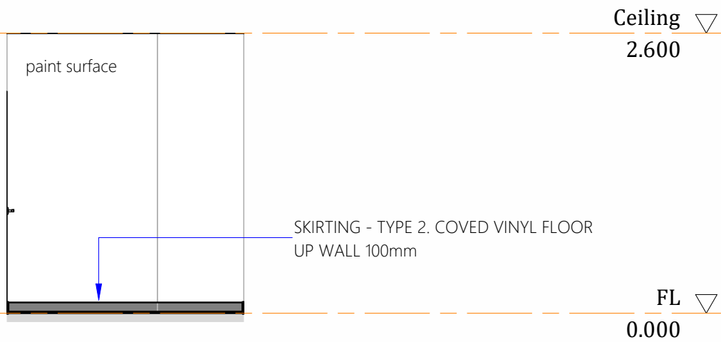
Elevation 4C 1 : 50
