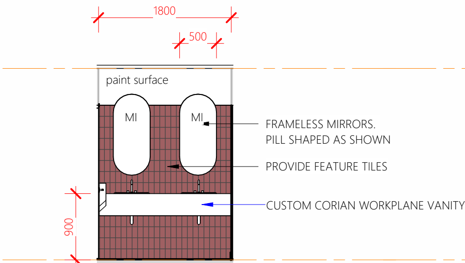
Elevation 4A 1 : 50
