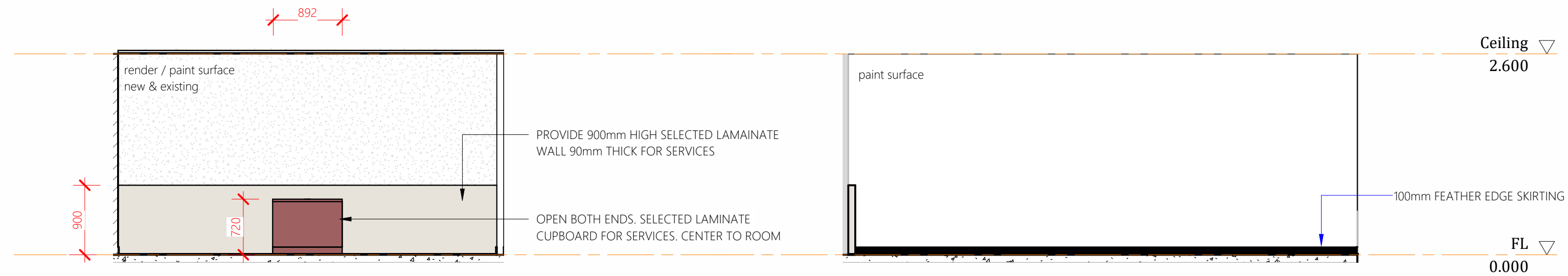
Elevation 5C 1 : 50
