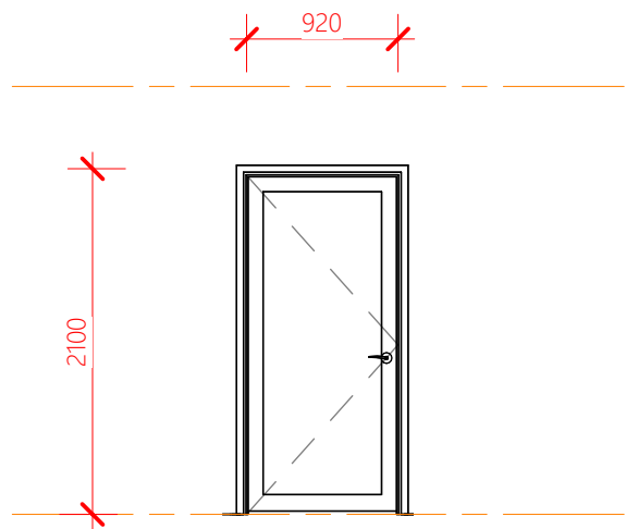
DOOR TYPE B
