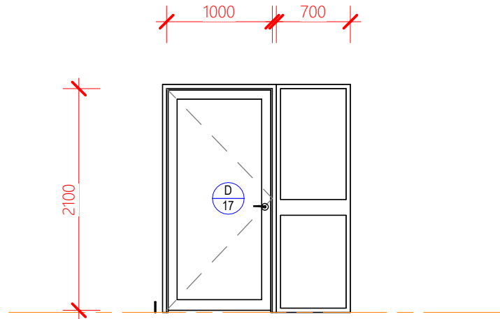
DOOR TYPE G
