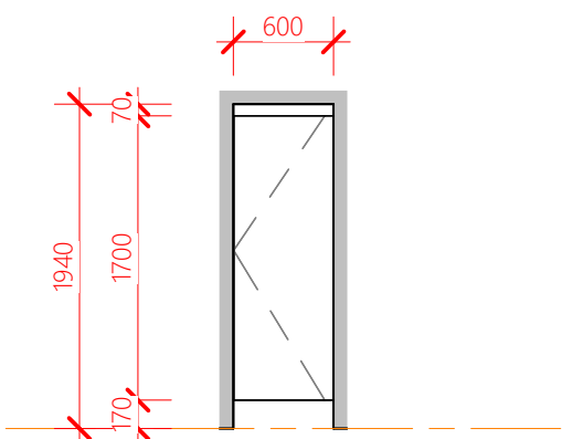
DOOR TYPE E
