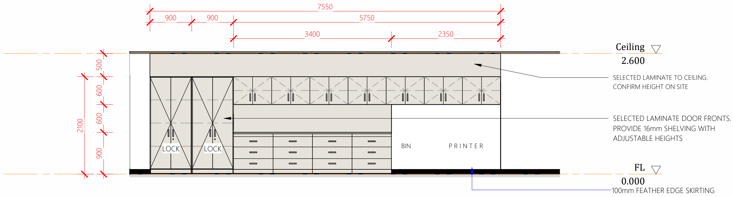
Elevation 2A
